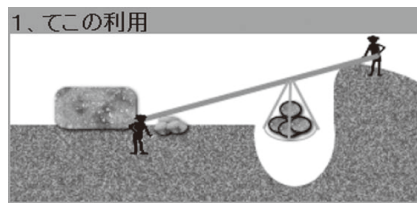
1、てこの利用 右の盛り土を下げると、石の重みで力が働いて、石が立ちます。
