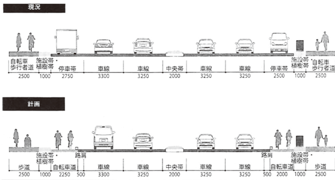
自転車通行空間(単路部)イメージ図(建設タイムズより)
