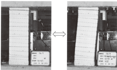
【SRF工法で補強した柱】
